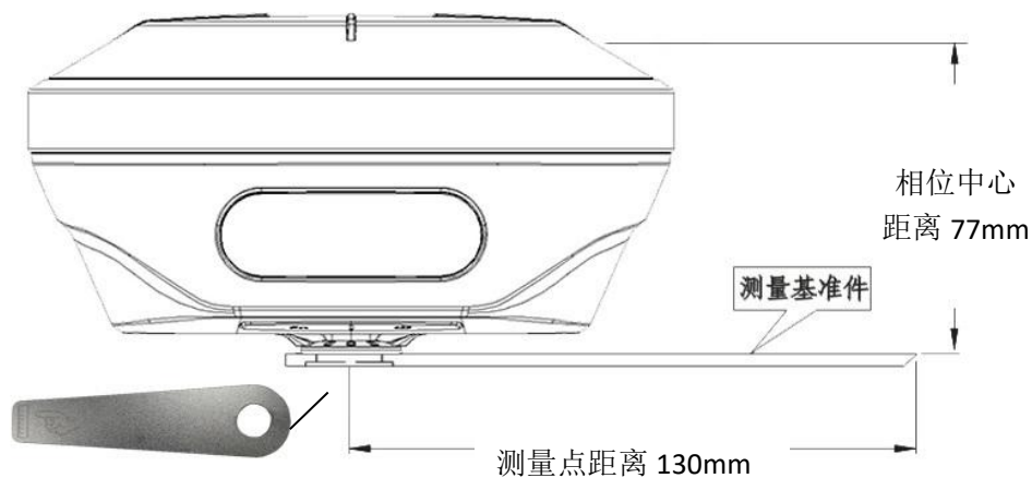
测量基准件
