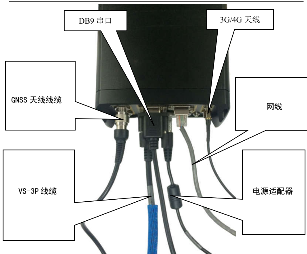
图 4-2 接收机连接图
